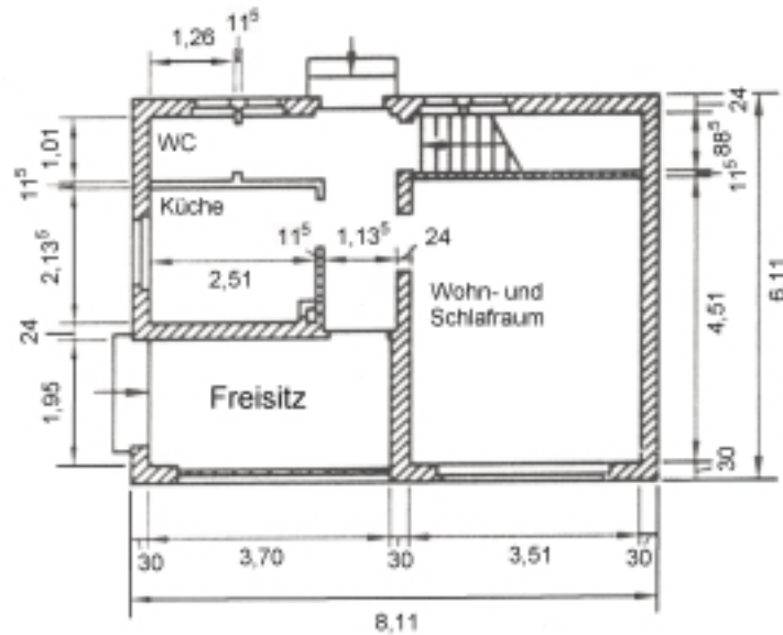
Erdgeschoss - Grundriss
