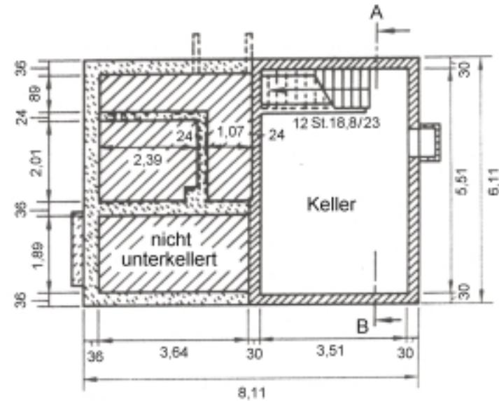
Kellergeschoss - Grundriss
