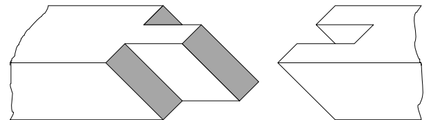
KARPFENSCHWANZ
