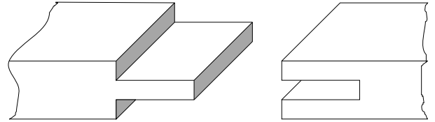
GERADER ZAPFEN
