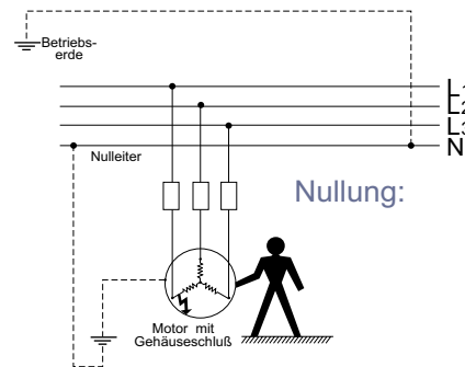
Schutz elektrischer Geräte vor Körperschluß
