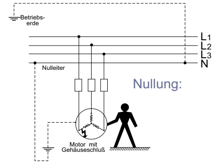
Schutz elektrischer Geräte vor Körperschluß
