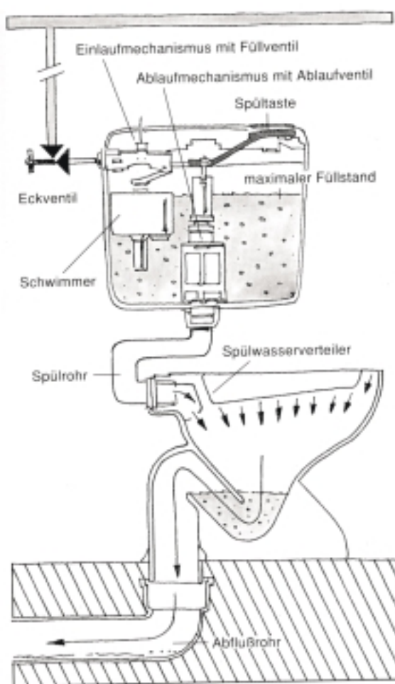
WC - Spülung
