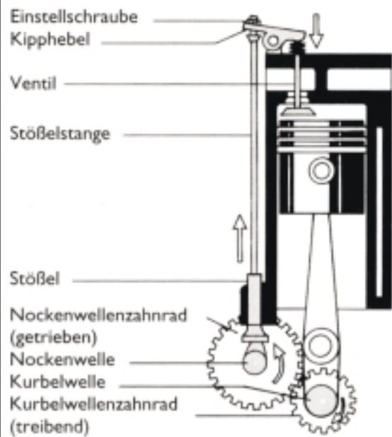
Motor - Ventile
