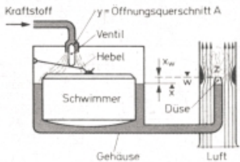
Vergaserfüllstand
